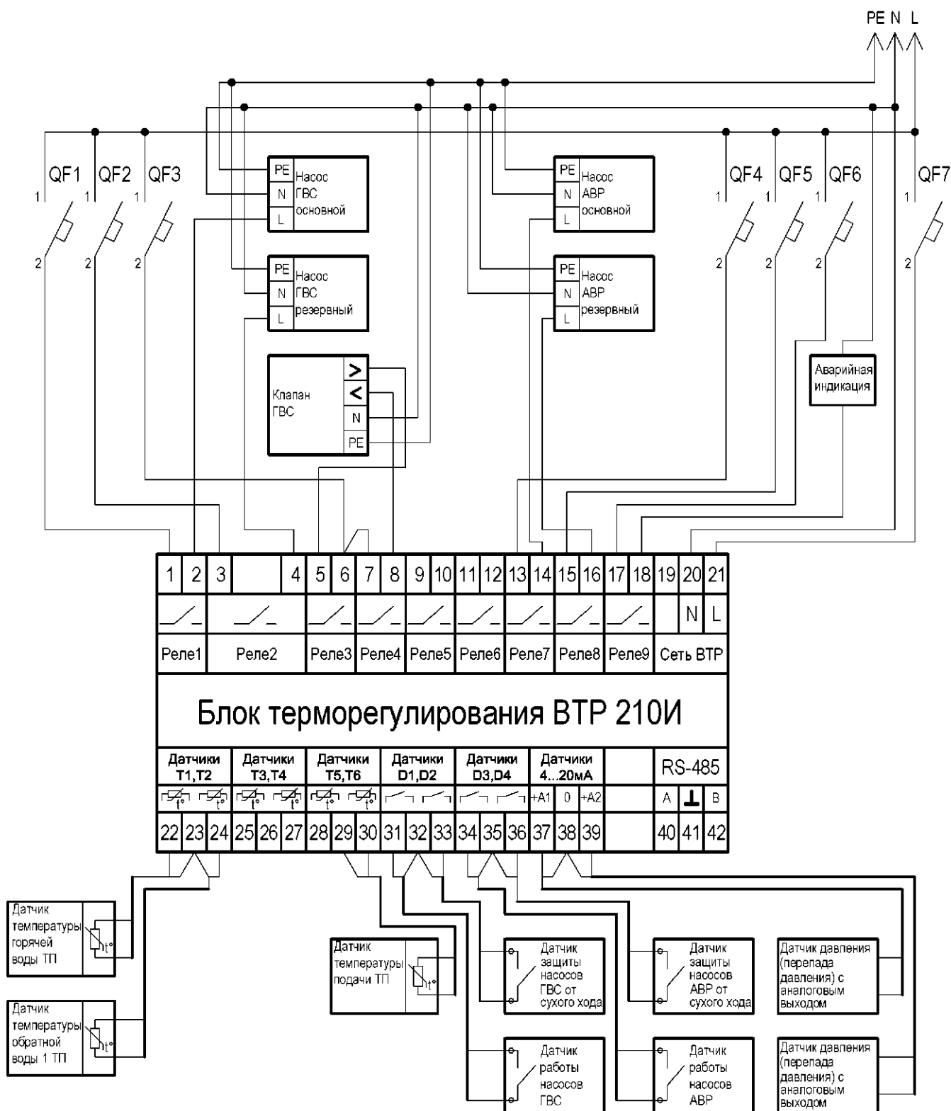
Рисунок В.9-Схема подключения регулятора ВТР 210И (программа 25) в системе управления контуром ГВС и контуром АВР насосов
