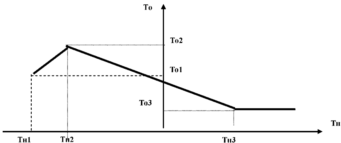
Рисунок 4.4 Вид графика To = f(T_{н})
