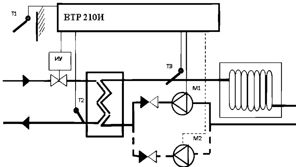
Рисунок Б.1 - Монтажная схема регулятора ВТР 210И (программа 10) в системе управления одним независимым контуром отопления
